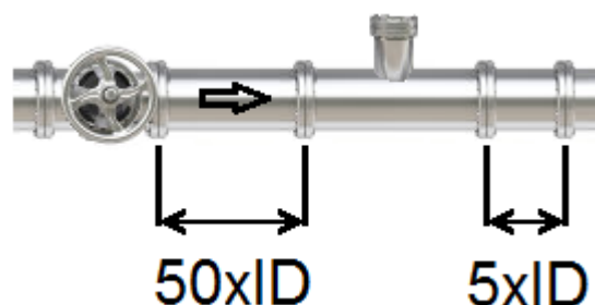
Valve – 50xID
